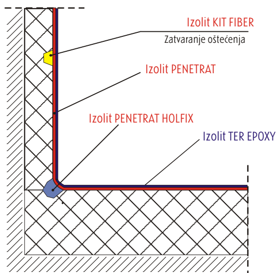
Detalj A
